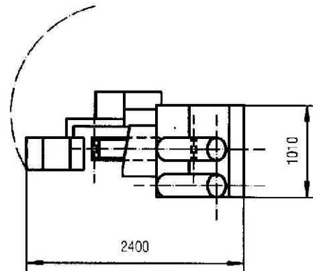
Draufsicht „A“ - topview „A“ - vue d'en haut „A“
